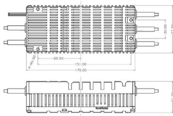
(b) ESC Dimensions
