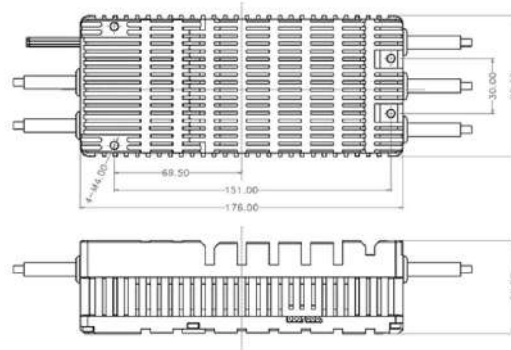
(b) ESC Dimensions
